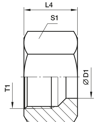
Überwurfmutter: M
